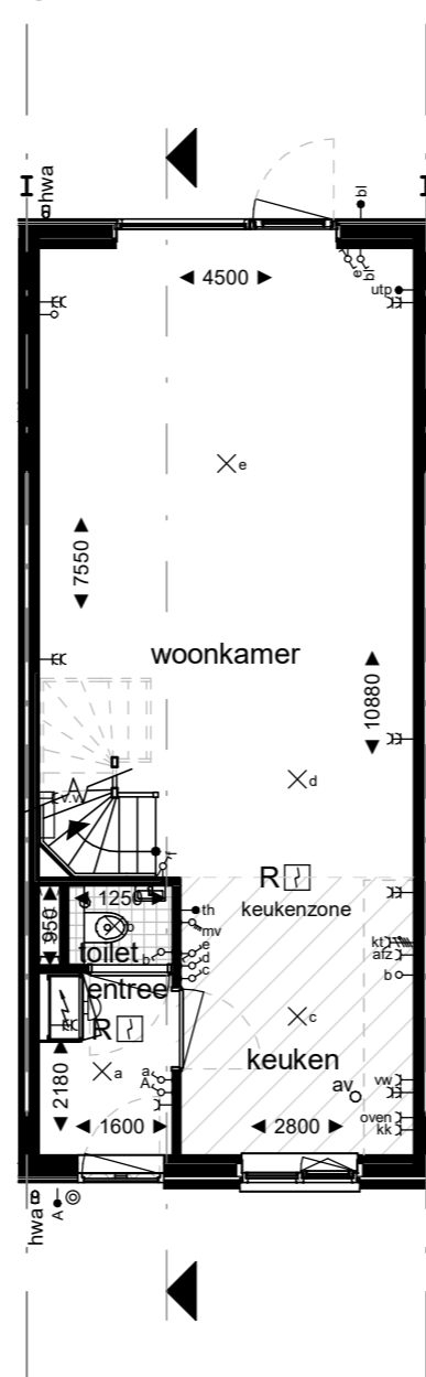
Begane grond: Optie uitbouw
