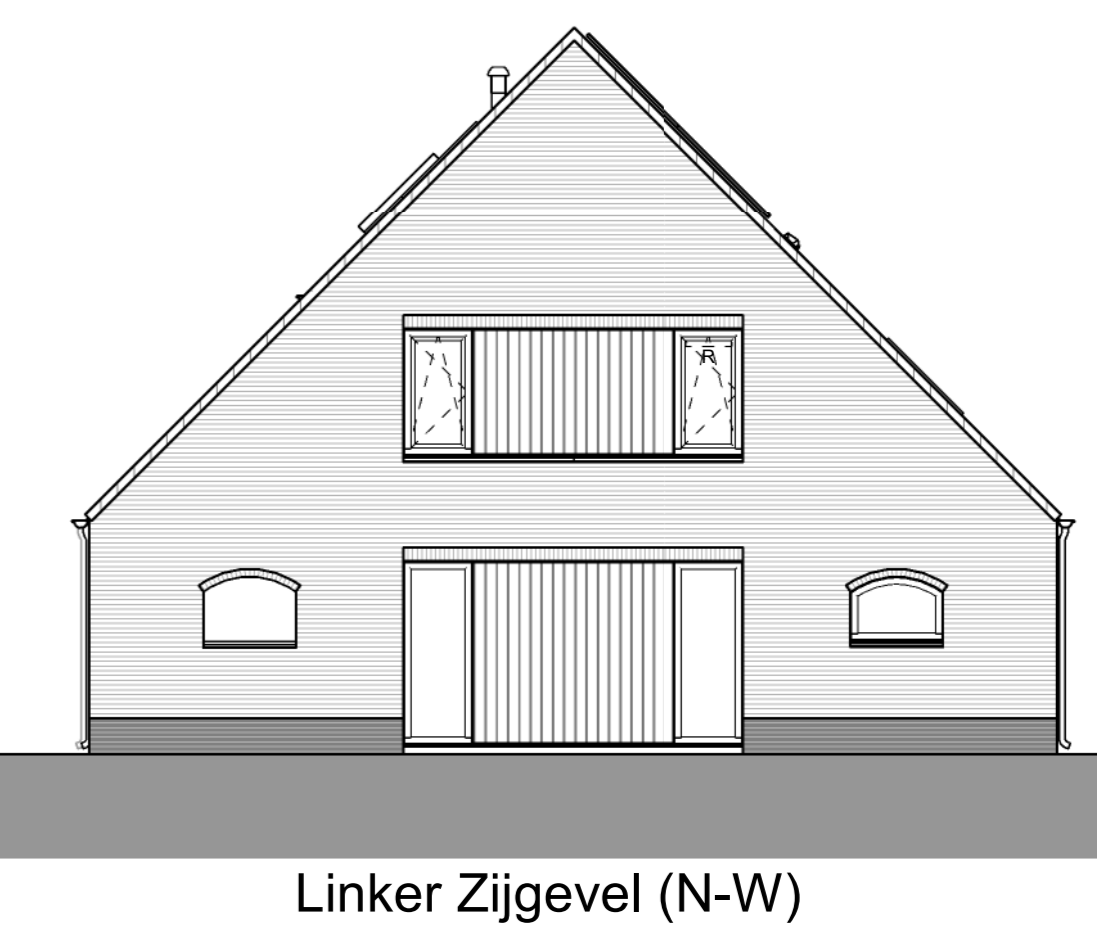
Linker Zijgevel (N-W)
