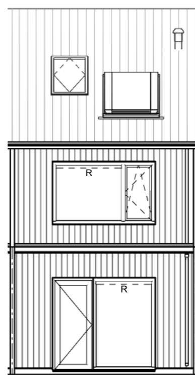
Achtergevel: Optie uitbouw
