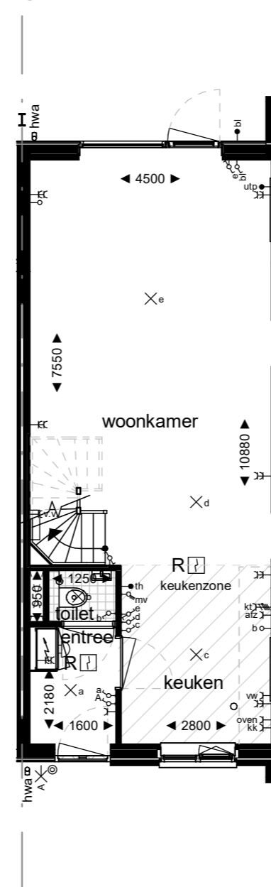
Begane grond: Optie uitbouw
