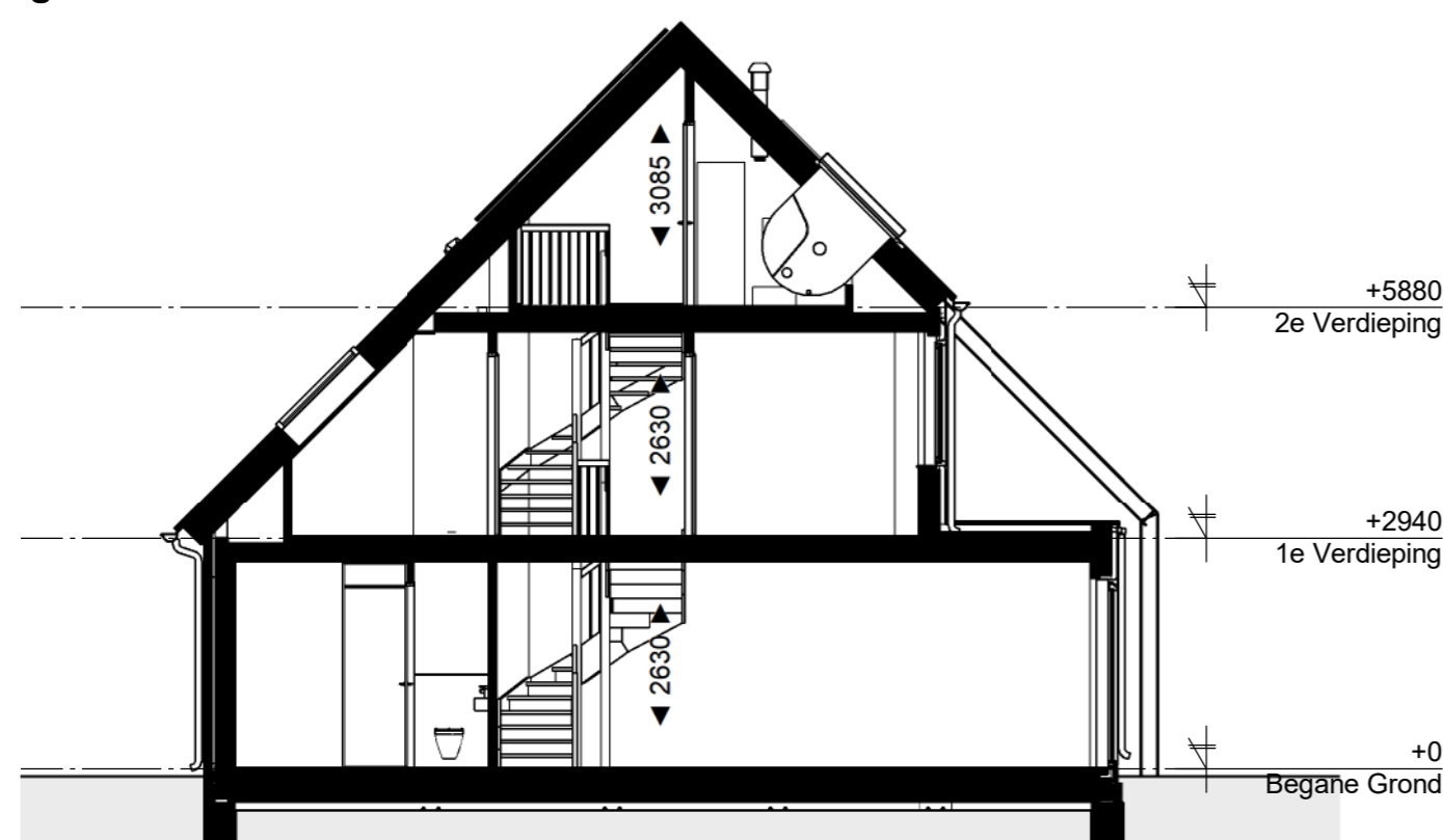
Doorsnede: Optie uitbouw
