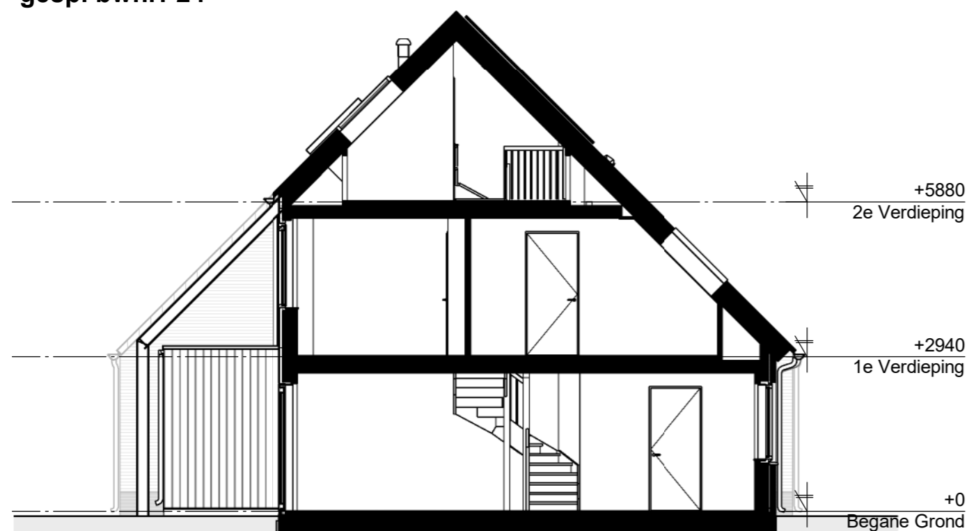
Zijgevel: Optie uitbouw
