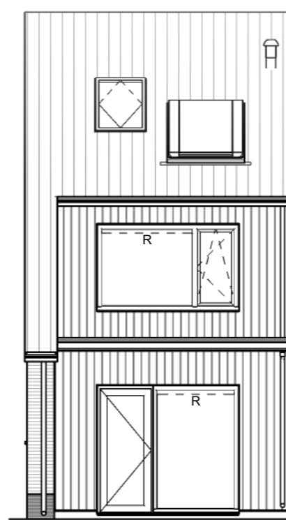
Achtergevel: Optie uitbouw
